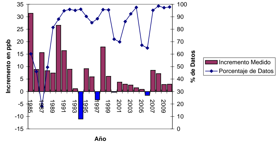
Incremento Anual de SF6 en Izaña
