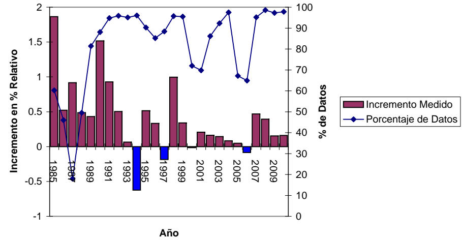
Incremento Anual de SF6 en Izaña
