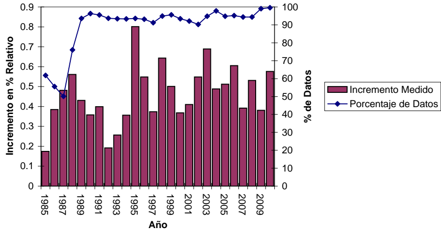
Incremento Anual de Óxido Nitroso en Izaña
